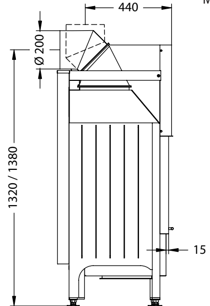
Seitenansicht M~1:20
