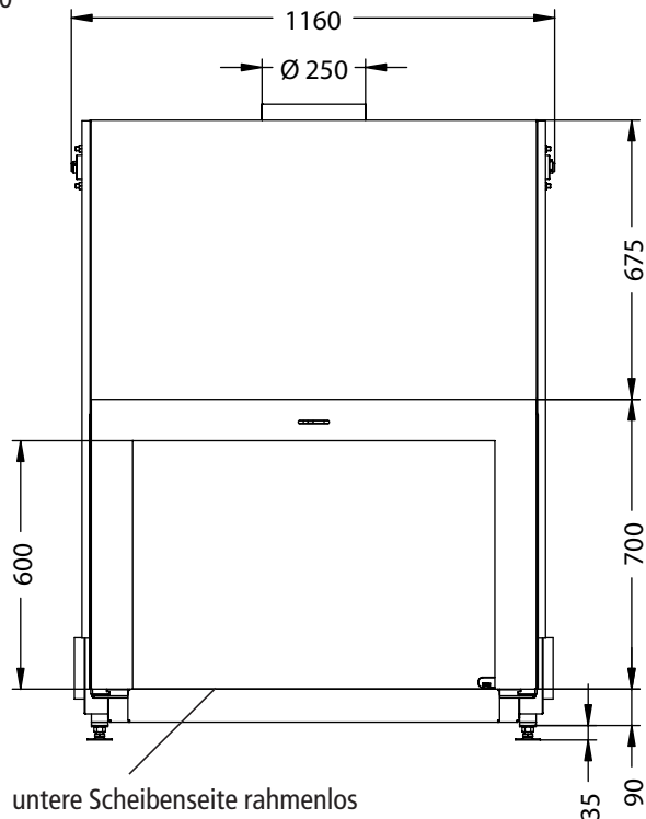
Vorderansicht M~1:20
